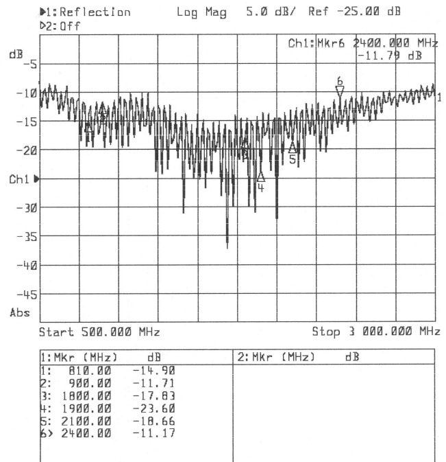
LOG MAG 500MHz – 3000MHz
