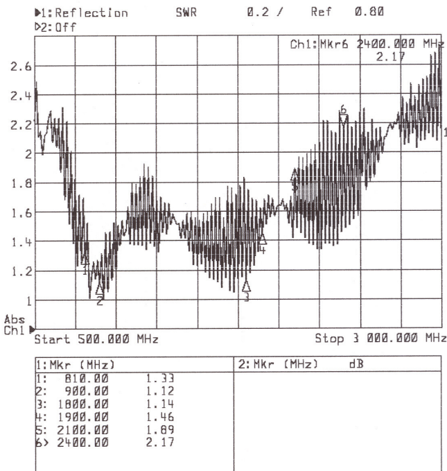
VSWR 500MHz – 3000MHz
