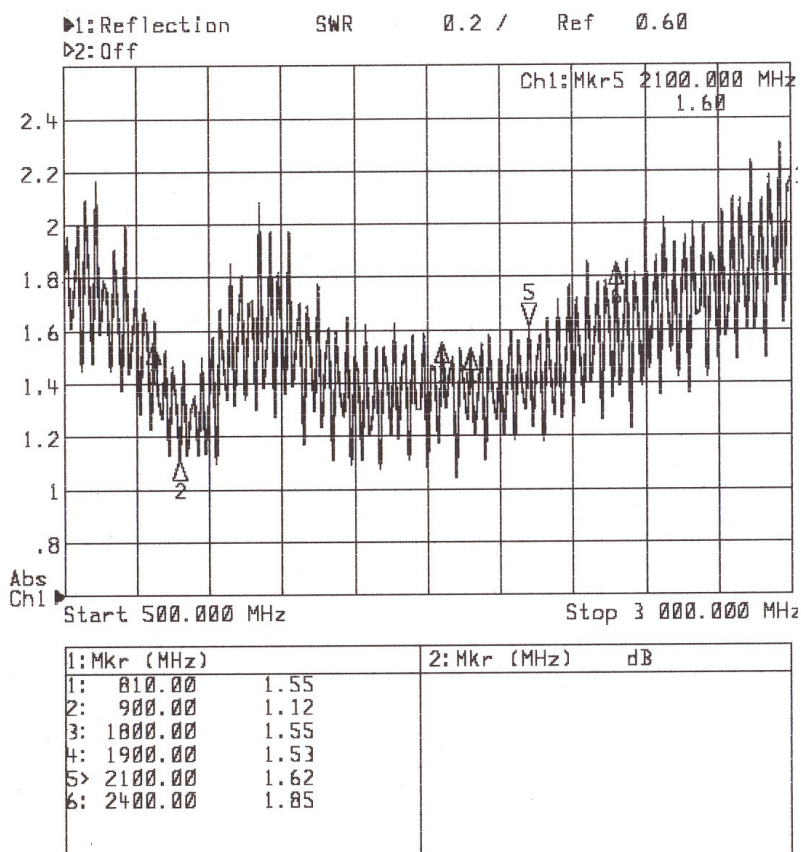
VSWR 500MHz – 3000MHz
